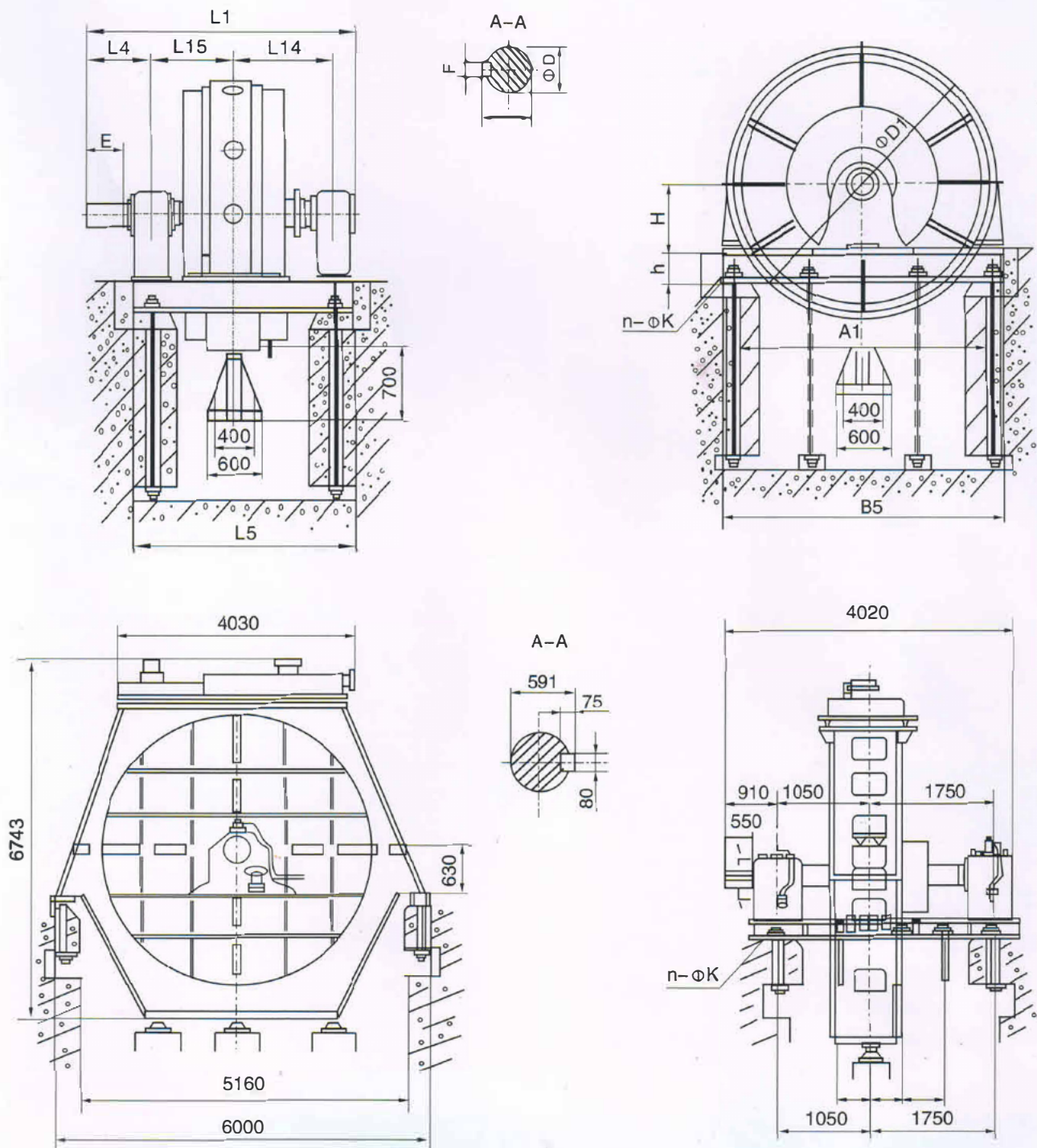
TDMK系列大型交流三相同步电动机外形图 TDMK series AC synchronous motor outline drawing
