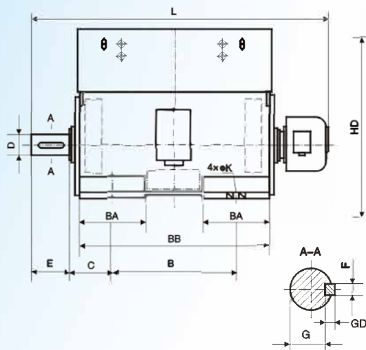
图1 YRKS400-500
