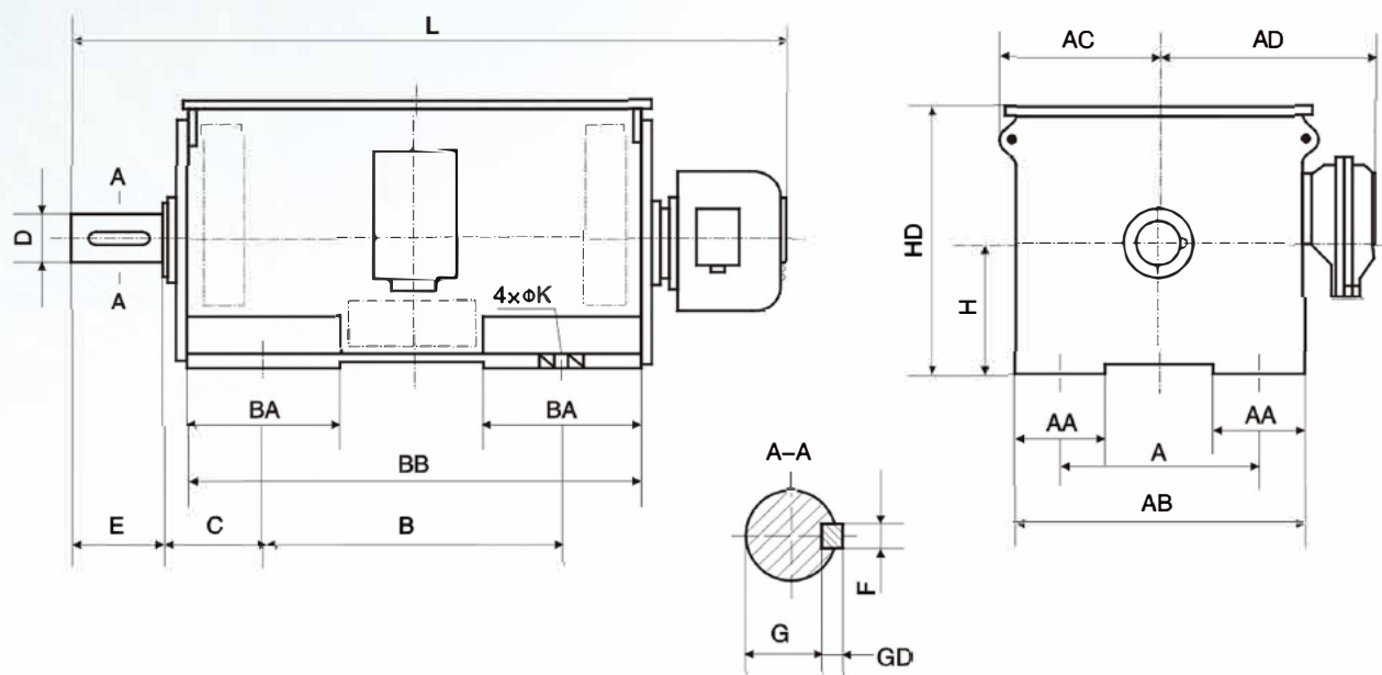
图1 YR355~450
