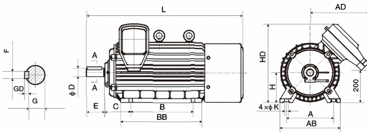
图 2 H450 ~ 560 外形图
